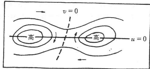
图 3 因经向风 v 的纬向非均匀性造成的副高带的断裂
